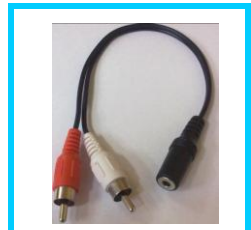
CAB-87(30) 音源線 (紅白公轉母) 30CM
