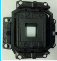
AMD-01 AMD底架
